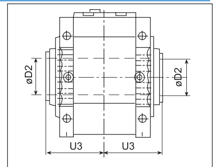
空心轴, 键连接, 具本尺寸见 49 页
